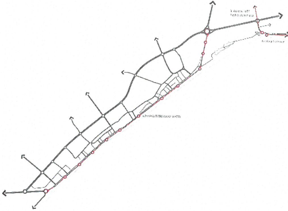
Şekil 5. Konyaaltı bölgesinde işletimine gerek duyulduğu durumda esnek tasarım müdahalesi ile sisteme entegre edilecek tramvay güzergahı ve durak noktaları.
