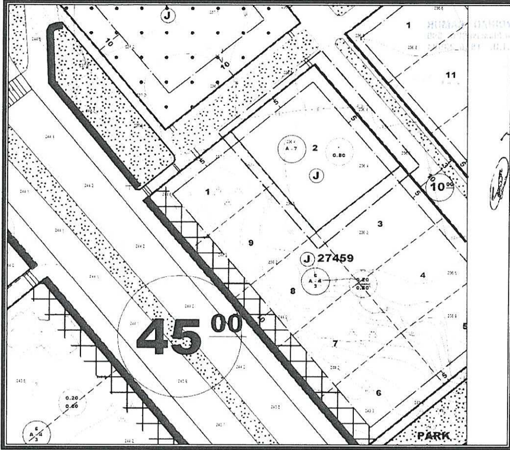
Şekil 4. Plan Örneği
