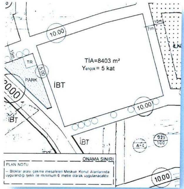
Mevcut ve Öneri 1/1000 Ölçekli UİP(Ölçeksiz)
