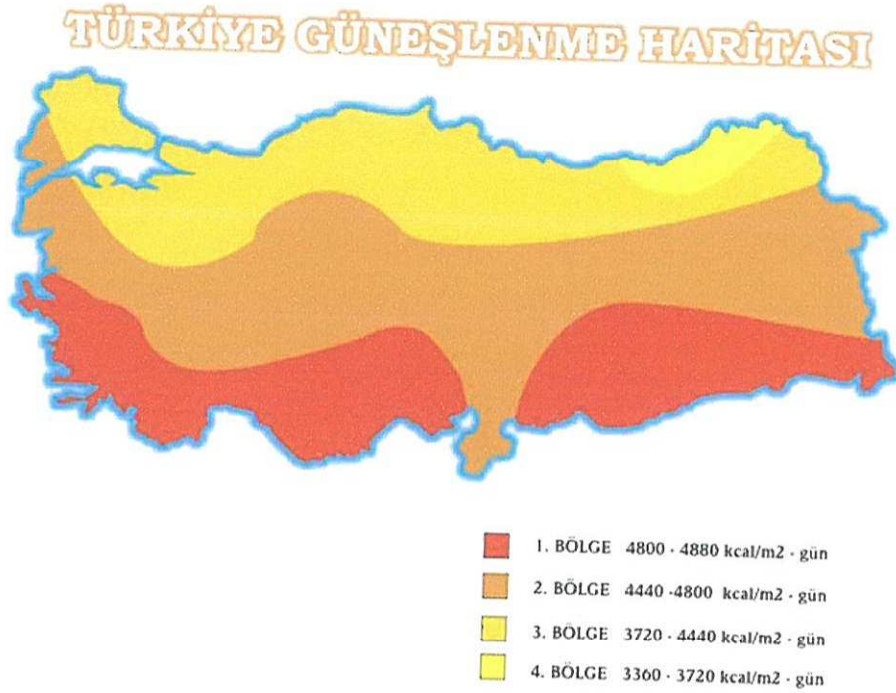
Şekil 2: Türkiye Güneşlenme Haritası
