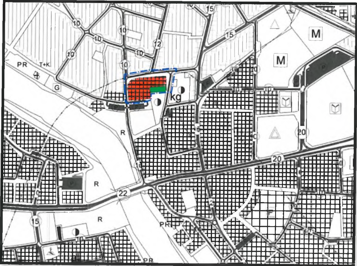
Şekil 4: Öneri Nazım İmar Planı Değişikliği
