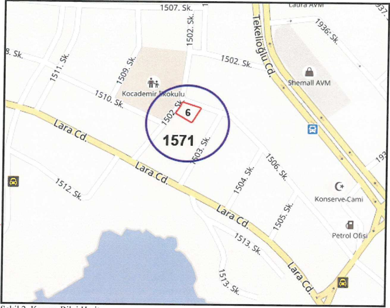
Şekil 2. Konum Bilgi Haritası
