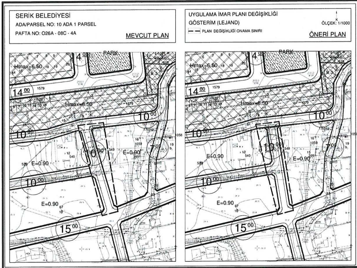
Şekil 5. Öneri 1/1000 Ölçekli Uygulama İmar Planı Değişikliği
