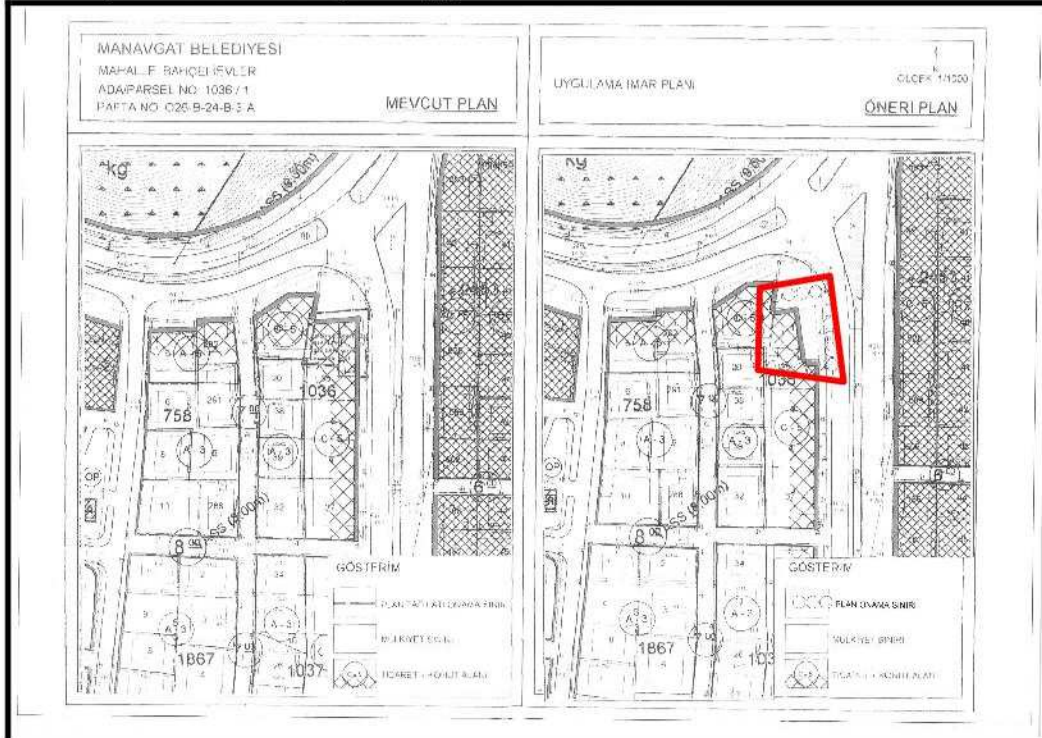
Şekil 3. 1/1000 Ölçekli Uygulama İmar Planı
