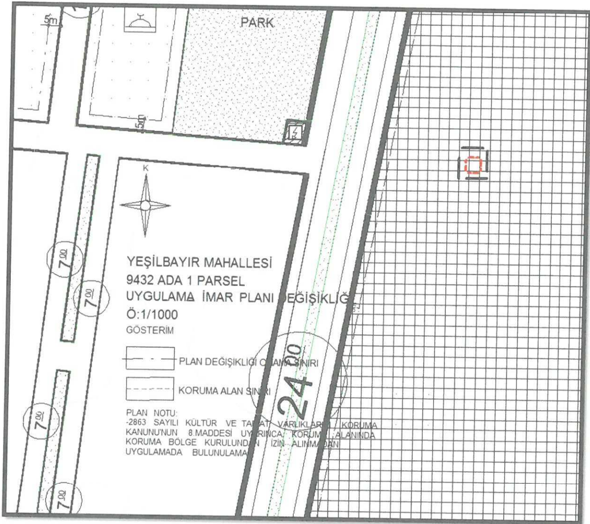
Şekil 5: Hazırlanan Öneri 1/1000 ölçekli Uygulama İmar Planı Görşeli.
