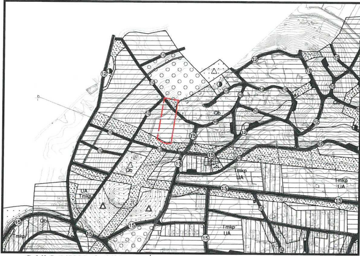
Şekil 5. 1/5000 ölçekli Nazım İmar Planı'ndaki Yeri
