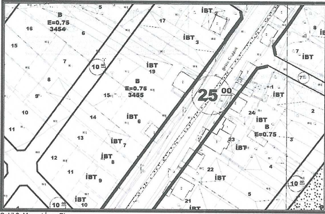
Şekil 6. Mevcut İmar Planı
