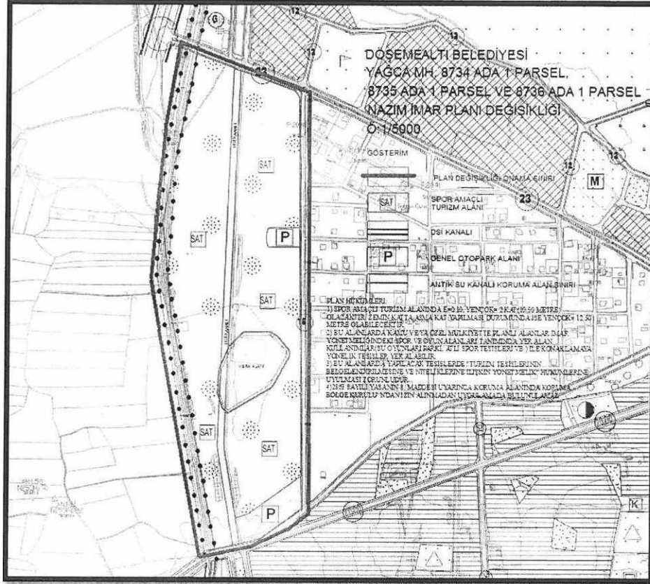
Şekil 6: Öneri 1/5000 ölçekli Nazım İmar Planı Görseli (Spor Amaçlı Turizm Alanı).
