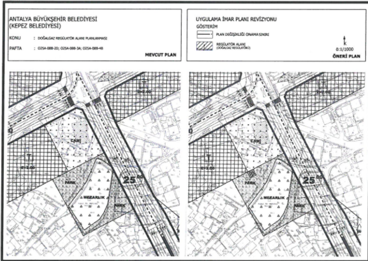
Şekil.2 1/1000 Uygulama İmar Plan Revizyonu (1. Bölge)
