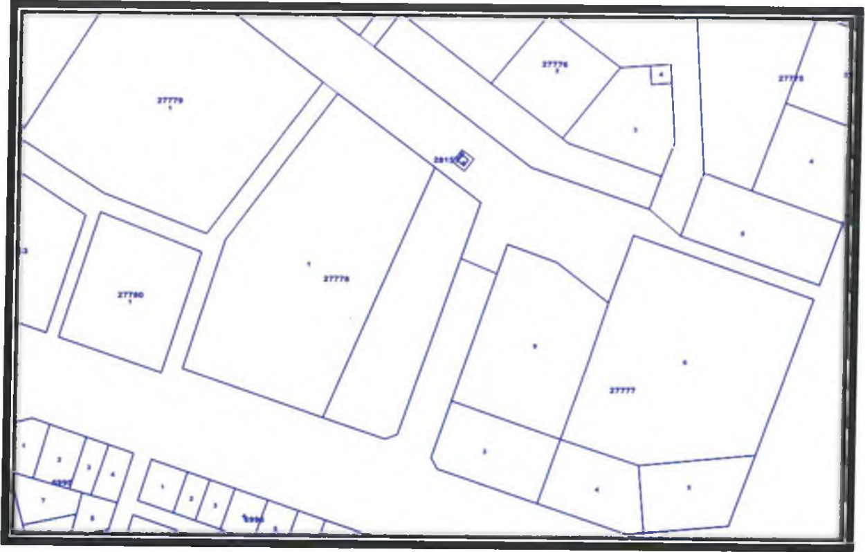
Şekil 4. Kadastral Durum
