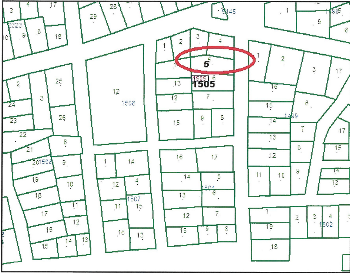
Şekil 5. Kadastral durum
