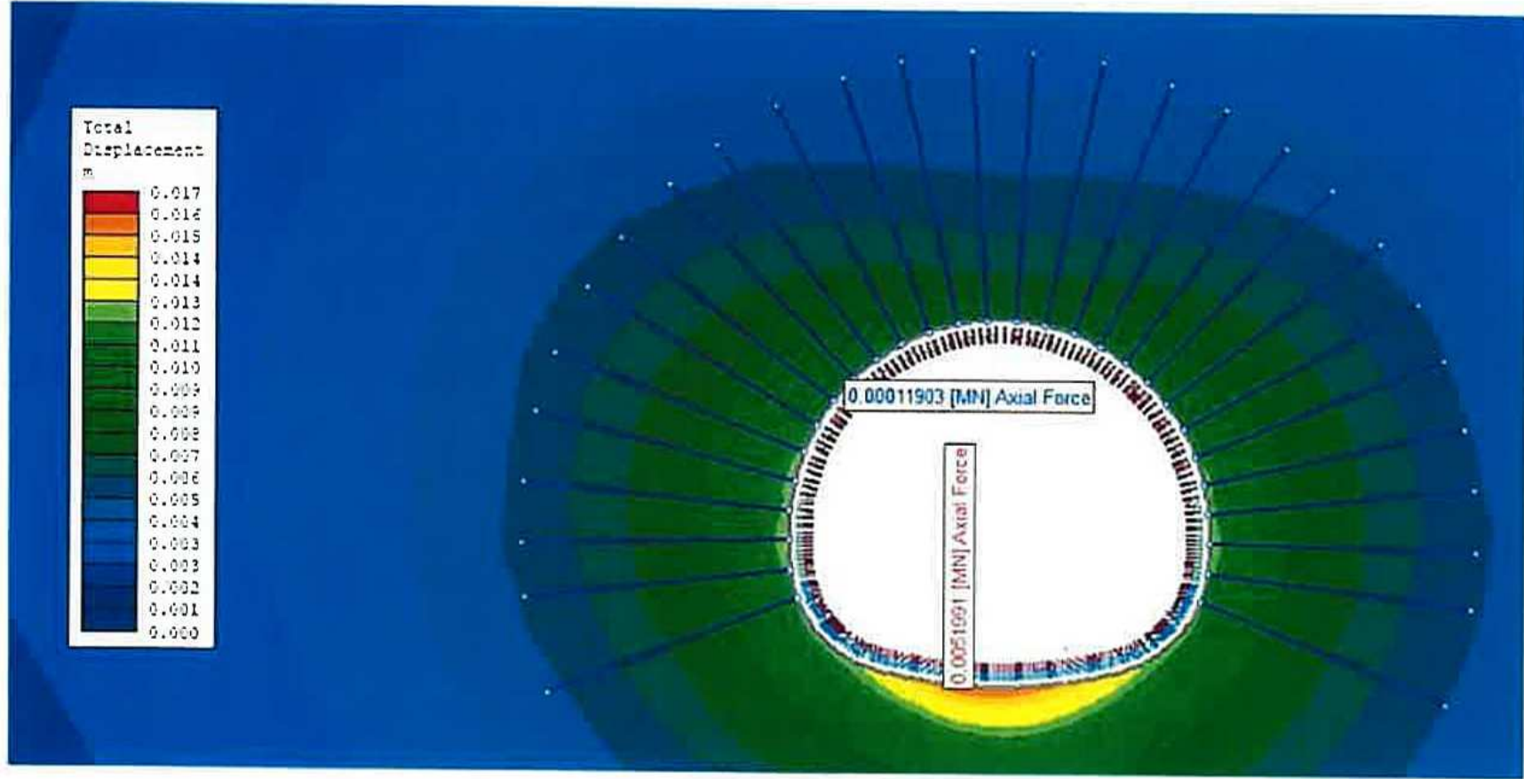
Şekil 4-7: Durum 2; Santral yapısı tünel inşaatından önce yapılması durumu
