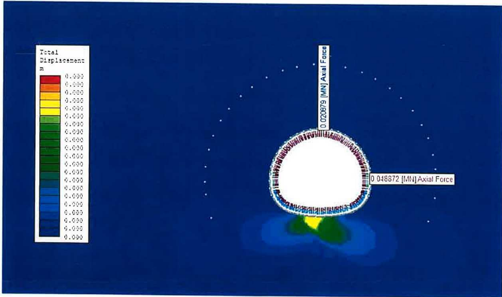
Şekil 4-8: Durum 3; Santral yapısının tünel inşaatından sonra yapılması durumu
