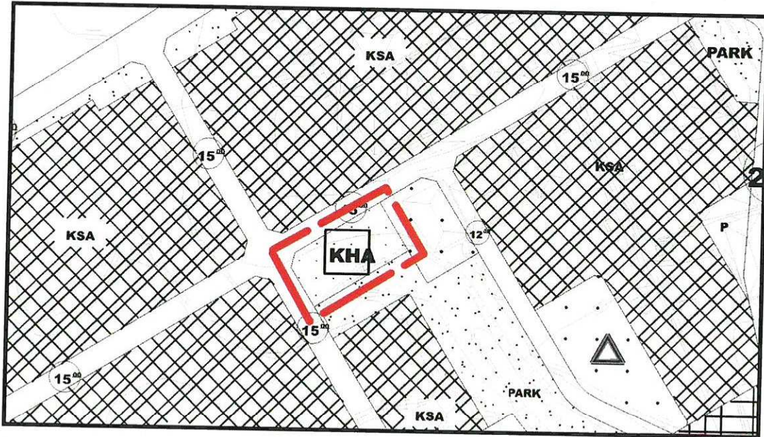
Resim 3: Öneri 1/1000 Ölçekli Uygulama İmar Planı Revizyonu Önerisi
